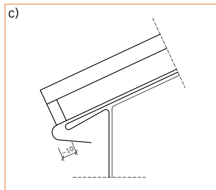
Rys. 18. Sposoby zakończeń rąbka: a) wersja zaokrąglona; b) wersja prosta c) wersja prostopadła
