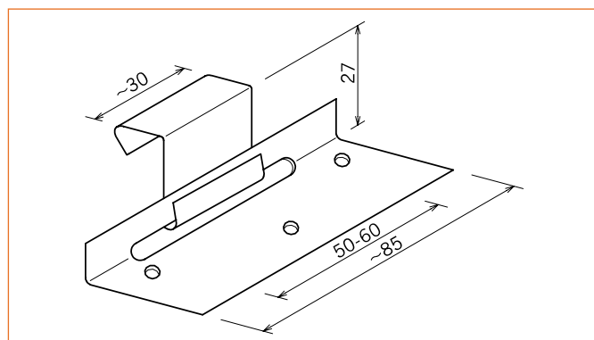
Rys. 16. Rodzaje haftek:
