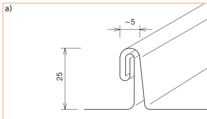
Rys. 15. Schemat połączenia rąbkowego stojącego:
