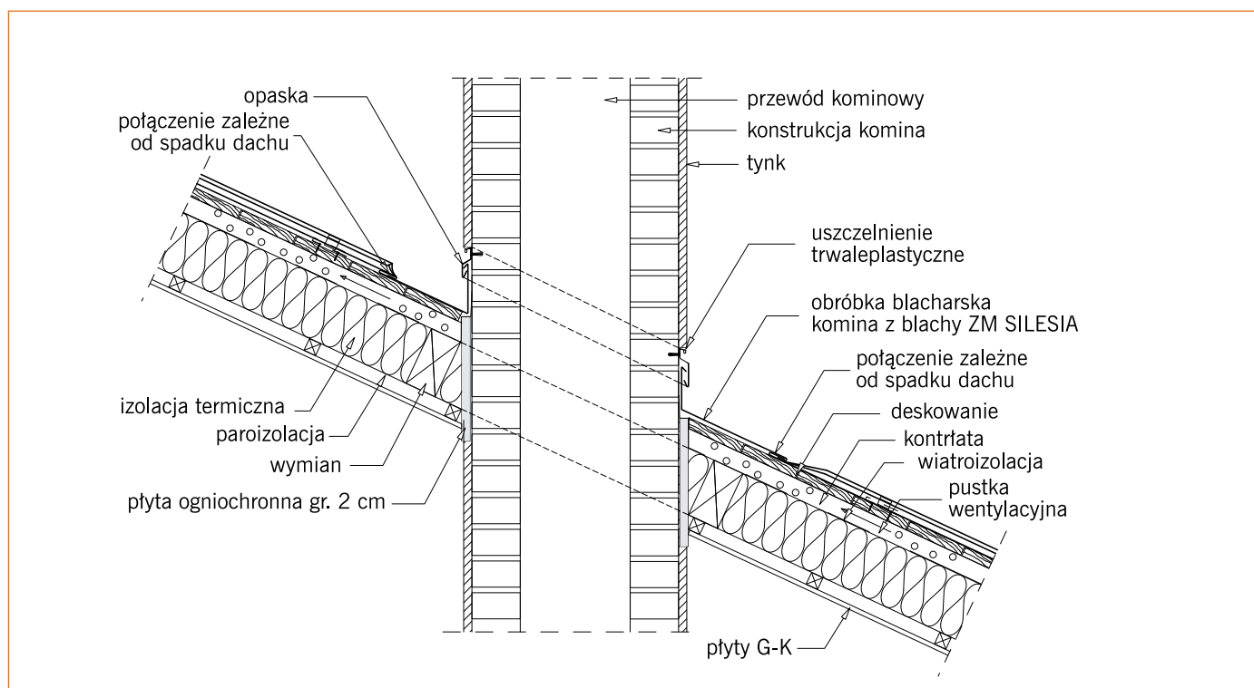
Rys. 8. Obróbka kominu
